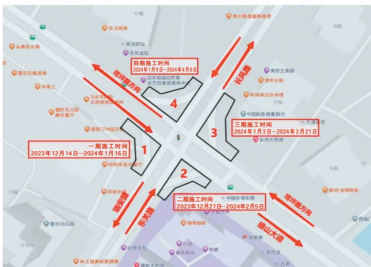
施工位置示意图 区公安局交巡警支队供图
